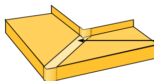
Eckverbindung Außenecke
