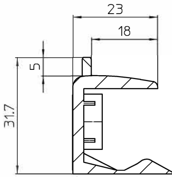
Schnitt Seitenabschluss Maßstab 1:1
