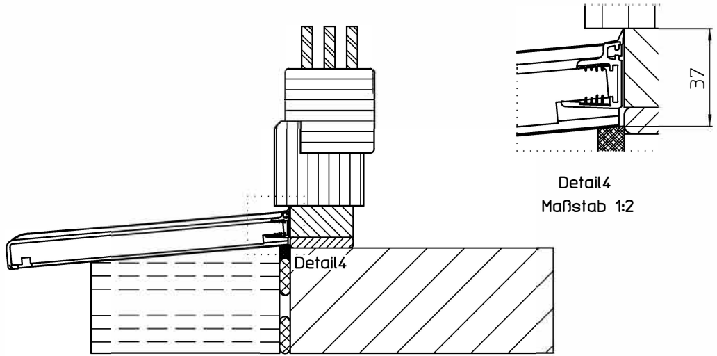
helopal contact mit Putzanschluss
