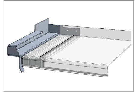
SlideAlu Wandeinschluss Fensterbank mit Ausklinkung und Hochzug
