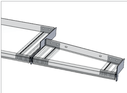
SlideAlu Kombi und SlideAlu L für schräge Laibung
