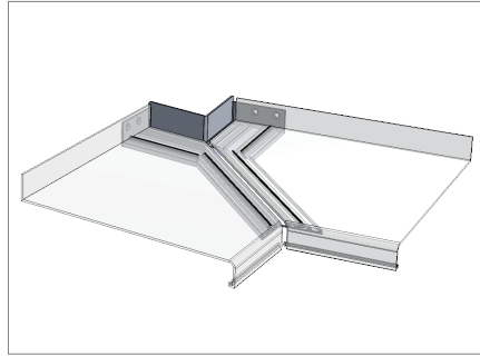
SlideAlu Y für Säule im Inneneck
