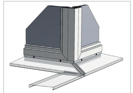
SlideAlu Eckeinbindung
