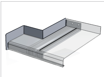
SlideAlu-L mit Ausklinkung hinten
