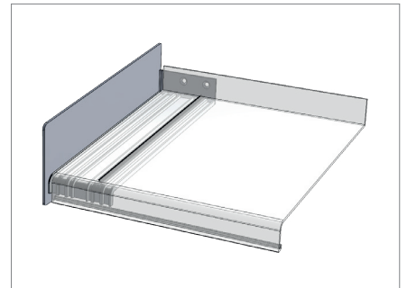
SlideAlu-L mit erhöhter Seitenwand
