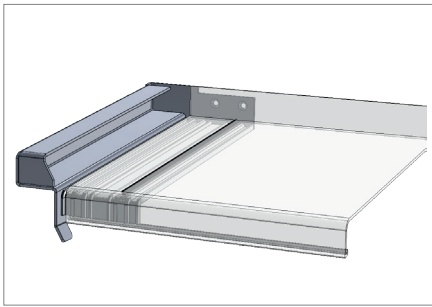
SlideAlu Wandanschluss Fensterbank
